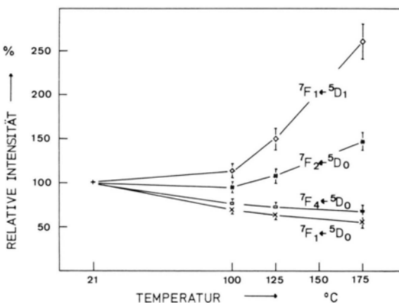
Abb. 2. Relative Intensitäten der Fluoreszenzübergänge von \text{Eu}^{3+} in wäßriger Lösung in Abhängigkeit von der Temperatur. (Intensität bei 21 °C = 100% für den jeweiligen Übergang.)
