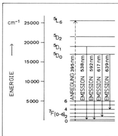
Abb. 1. Partielles Therschema von \text{Eu}^{3+} , Energiewerte aus Carnall et al. [6].
